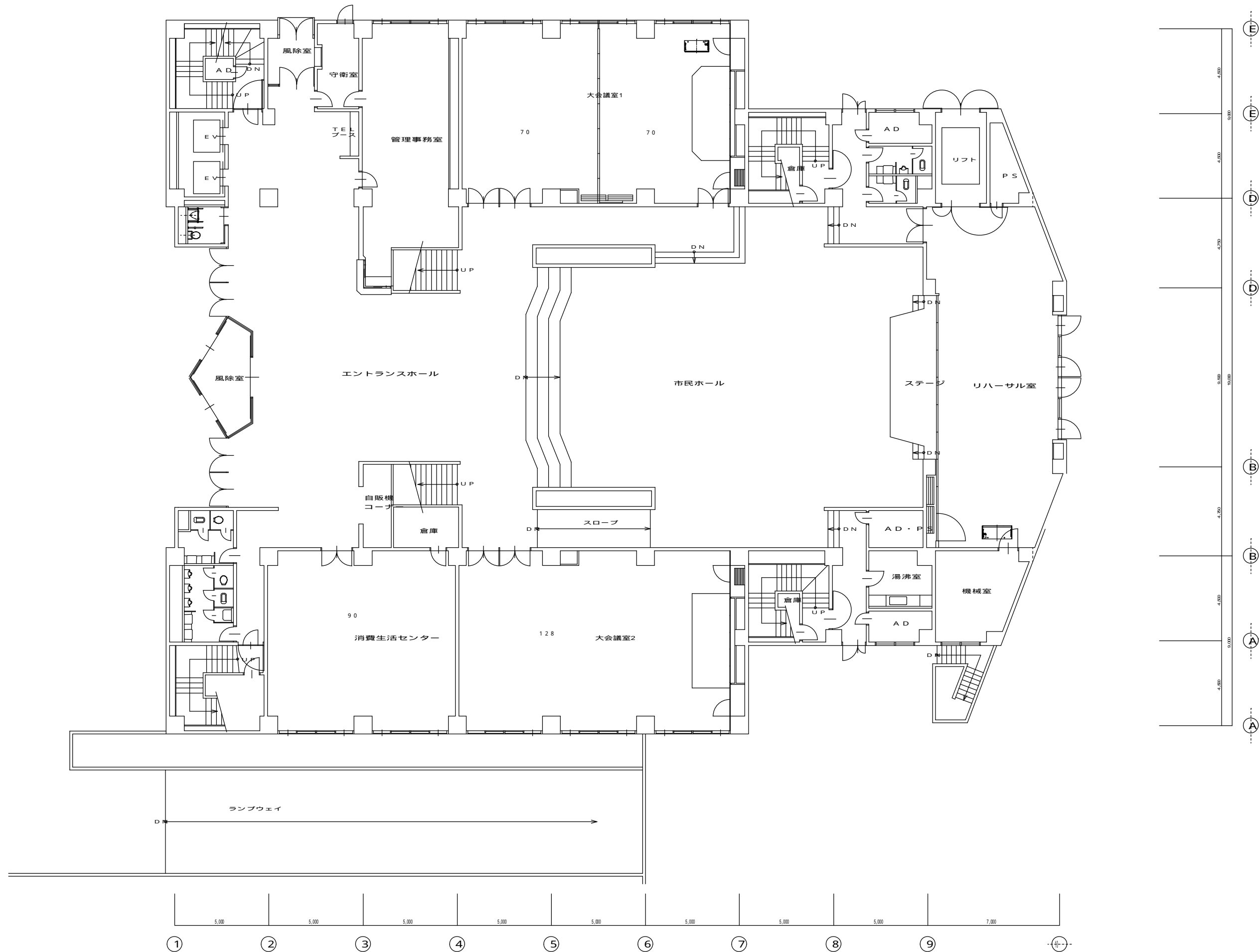
1階平面図 1 : 100
