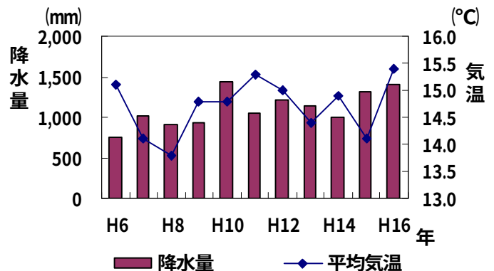
図1-2 降水量と平均気温の変化
