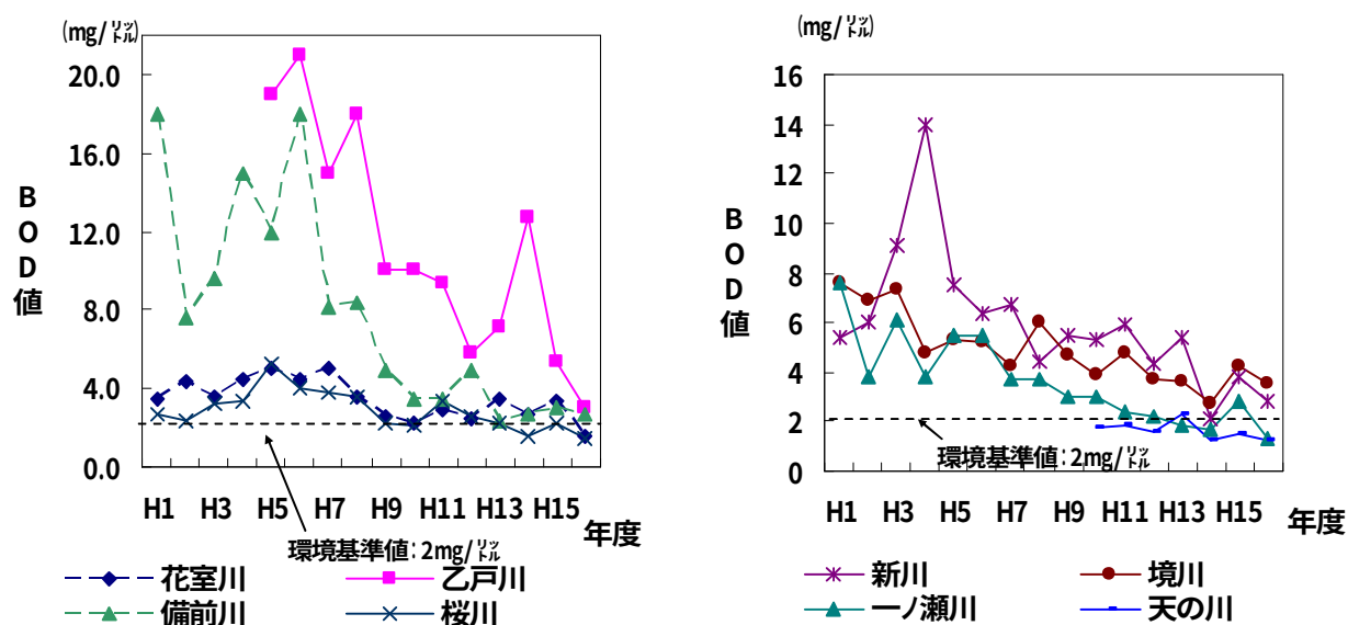
図4-1-4 河川のBOD値の変化
