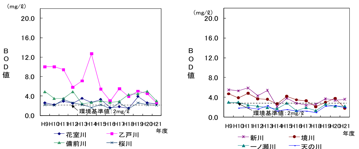
図4-1-4 河川のBOD値の変化
