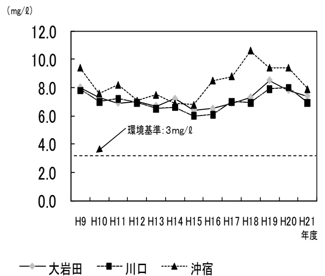
図4-1-3 霞ヶ浦の土浦沿岸のCODの変化
