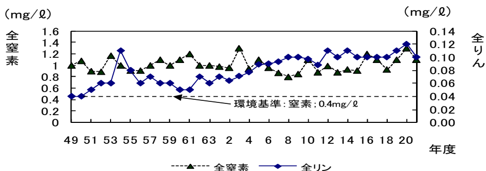
図4-1-2 霞ヶ浦の栄養塩の濃度変化
