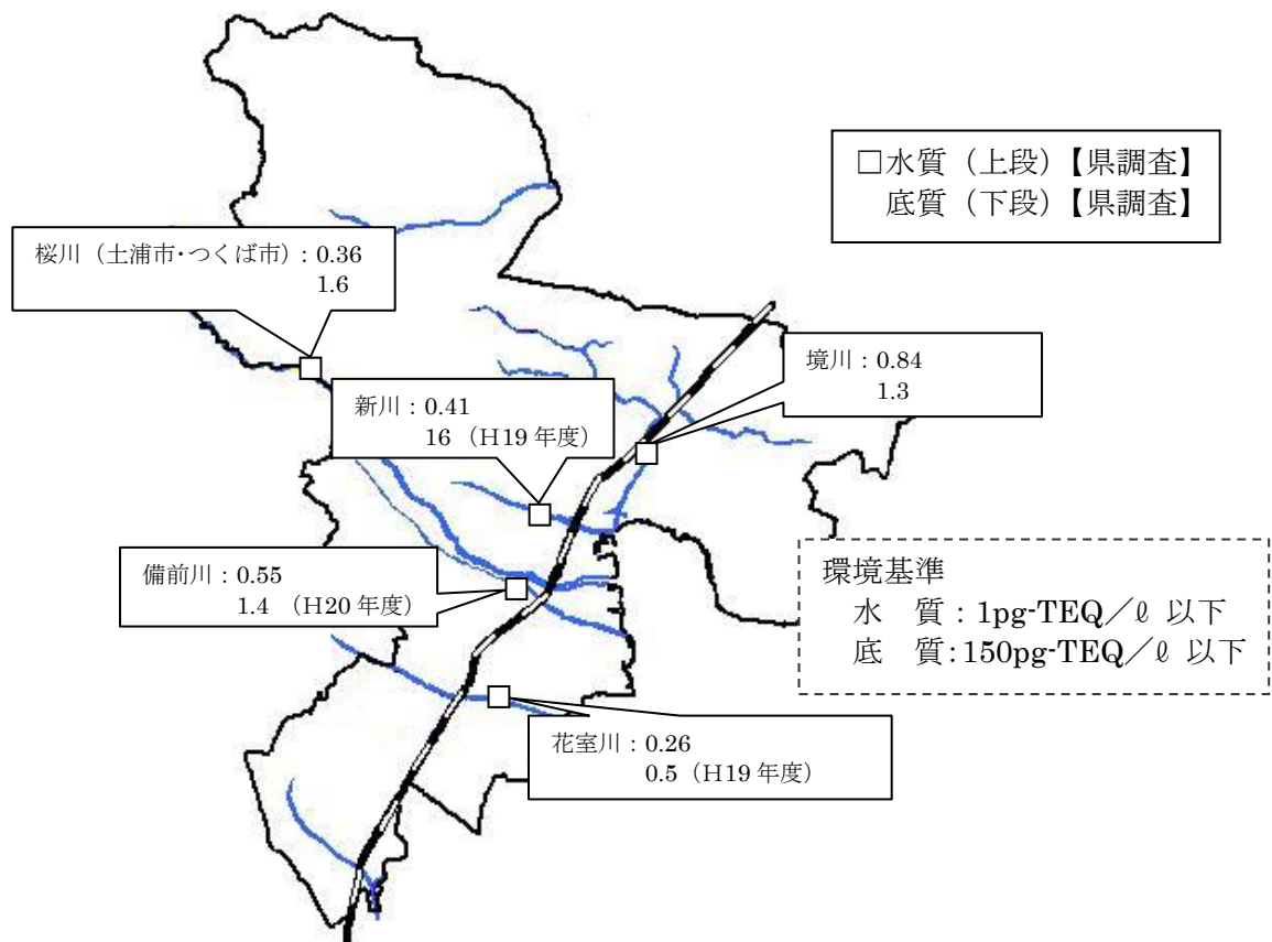
図4-2-7 平成21年度 公共用水域の水質・底質に係るダイオキシン類調査結果
