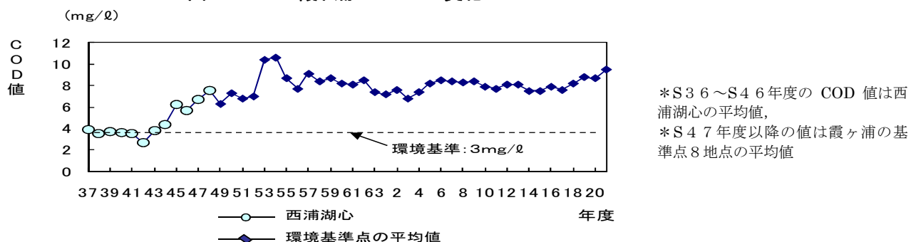
図4-1-1 霞ヶ浦のCODの変化
