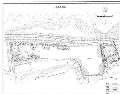
(仮称) 赤池公園計画平面図
