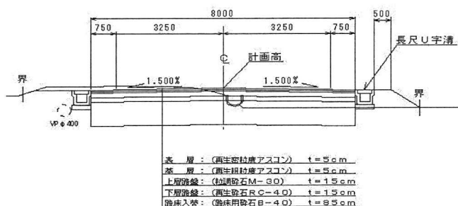
標準横断面
