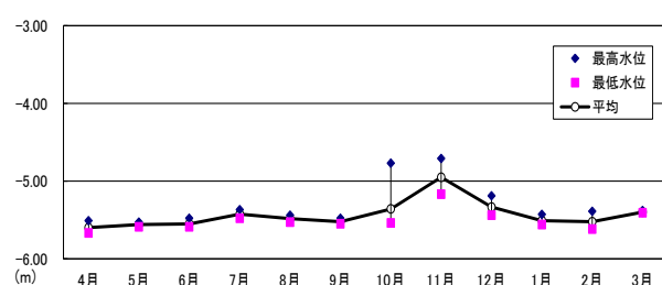
③天谷宅（神立町）の地下水位変動状況
