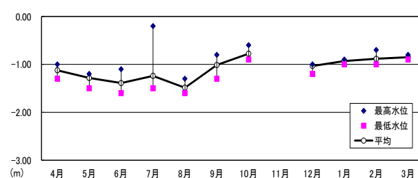
④太洋社（中央一丁目）の地下水位変動状況
