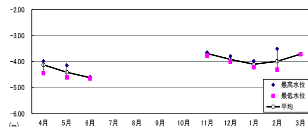
⑥荒川沖消防署（中荒川沖）の地下水位変動状況
