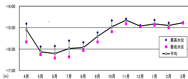
②皆藤宅（神立町）の地下水位変動状況
