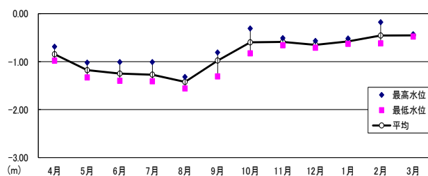
⑦桜児童遊園（桜町四丁目）の地下水位変動状況
