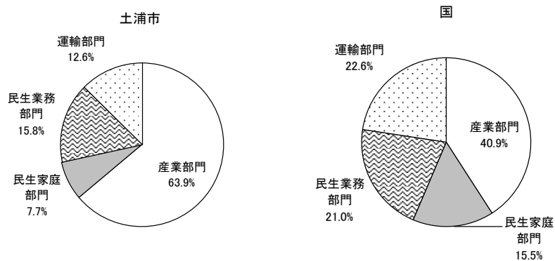
図 3-4-5 エネルギー起源 CO2 排出量の内訳と国との比較 (2005 年度)
