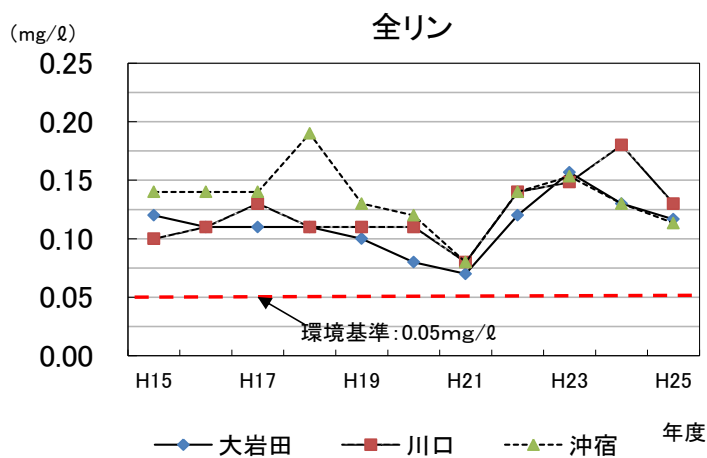
図 3-2-9 土浦沿岸の全リンの推移
