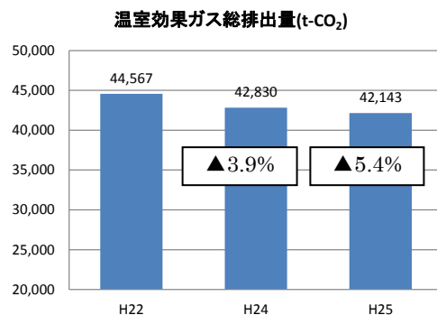
図 4-1-2 温室効果ガス総排出量実績
