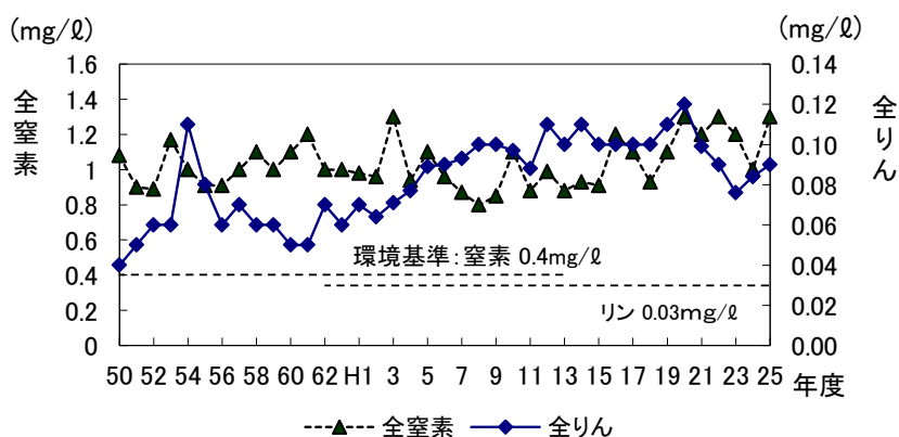
図 3-2-6 霞ヶ浦の全窒素と全りんの推移
