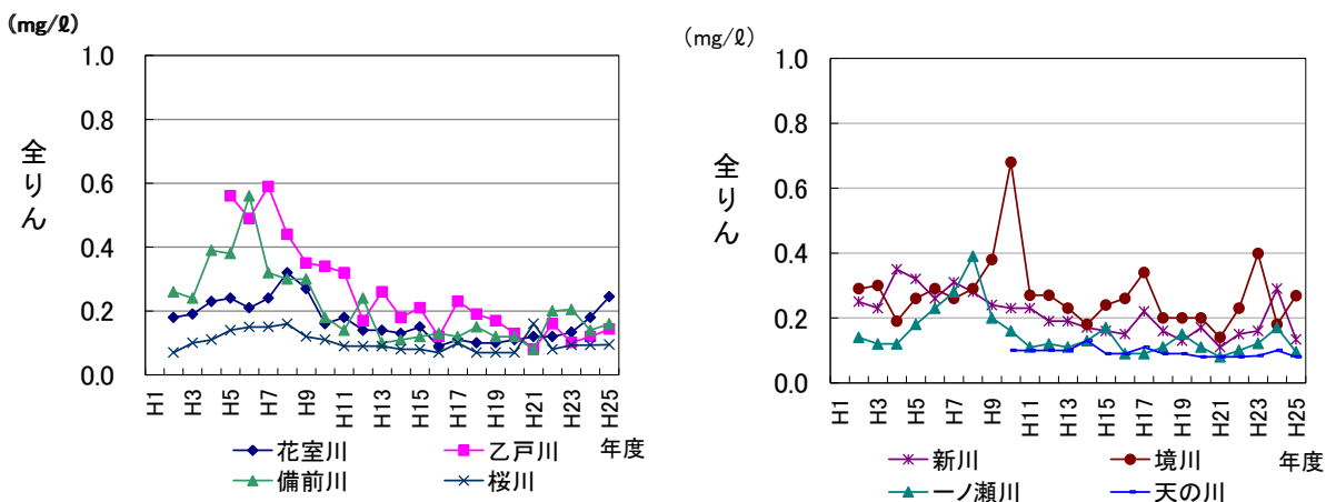
図 3-2-12 河川の全りんものの推移
