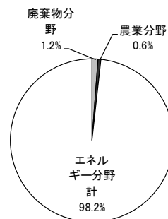
図 3-4-4 温室効果ガスの排出量の内訳
