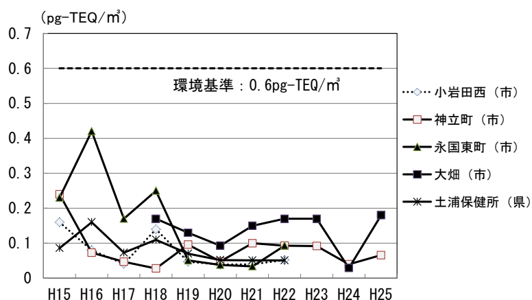
図 3-2-19 大気中のダイオキシン類測定結果
