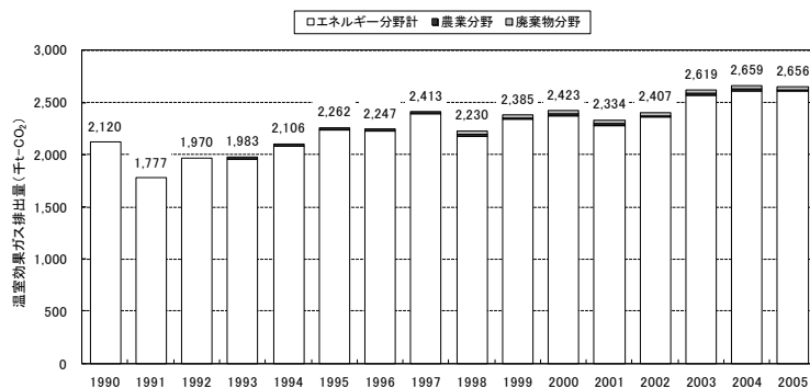
図 3-4-3 温室効果ガスの排出量の推移
