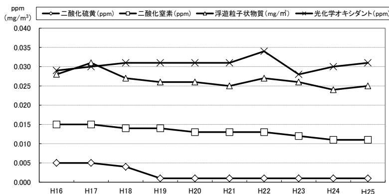
図 3-2-2 一般大気測定局における大気汚染物質（年平均値）
