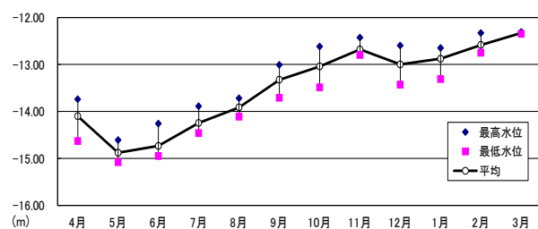
①中川宅（神立町）の地下水位変動状況
