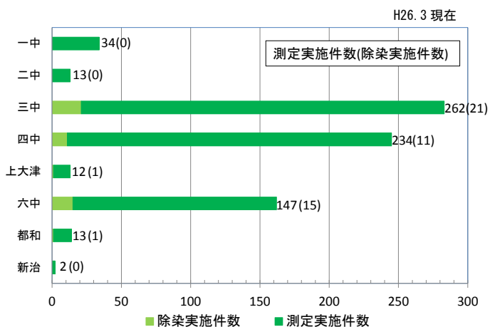
図 3-2-18 一般住宅の地区別放射線量測定及び除染実施状況
