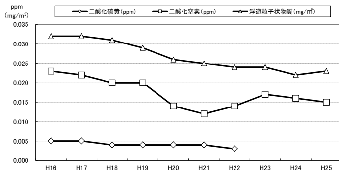
図 3-2-3 自動車排ガス測定局（中村）における大気汚染物質（年平均値）
