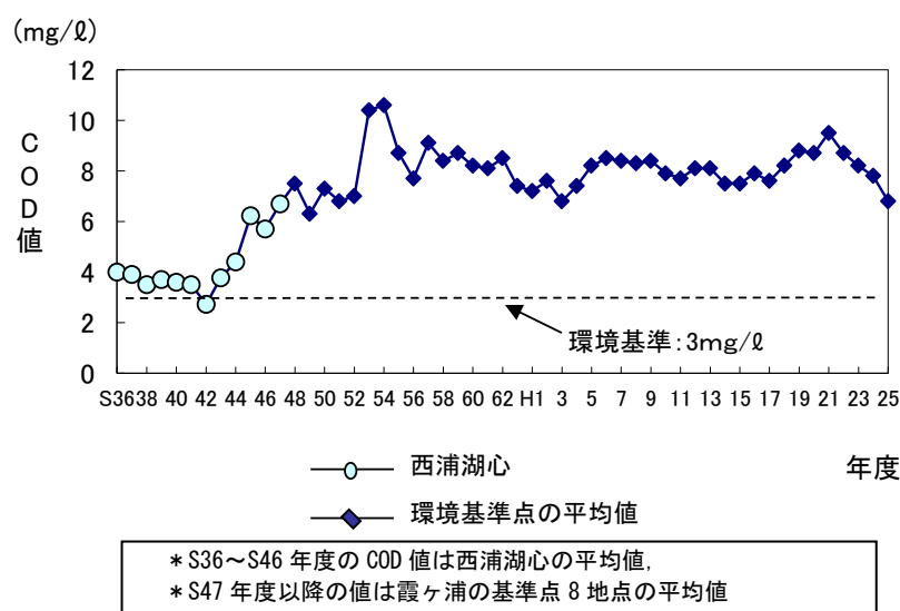
図 3-2-5 霞ヶ浦のCODの推移
