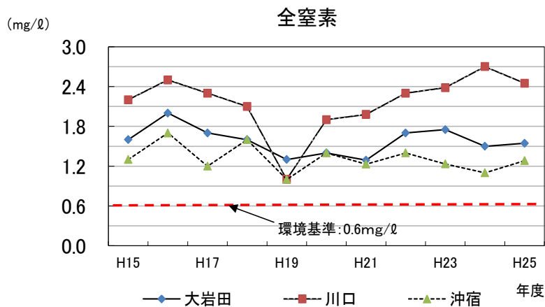
図 3-2-8 土浦沿岸の全窒素の推移
