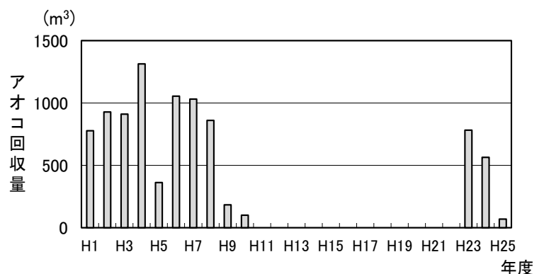
図 3-2-15 アオコ回収の実績
