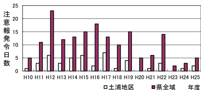
図 3-2-4 光化学スモッグ注意報発令状況
