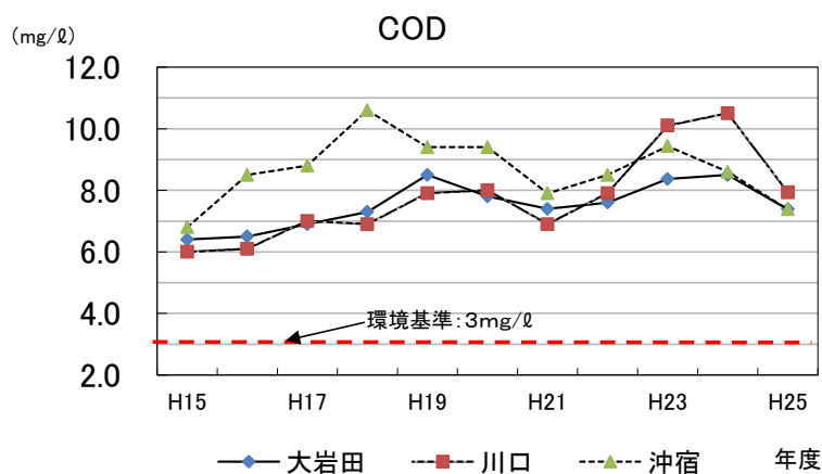
図 3-2-7 土浦沿岸のCODの推移
