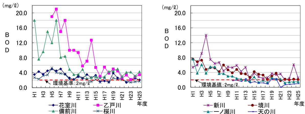
図 3-2-10 河川の BOD の推移
