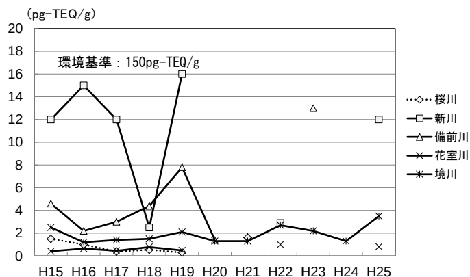
図 3-2-21 底質中のダイオキシン類測定結果（茨城県）
