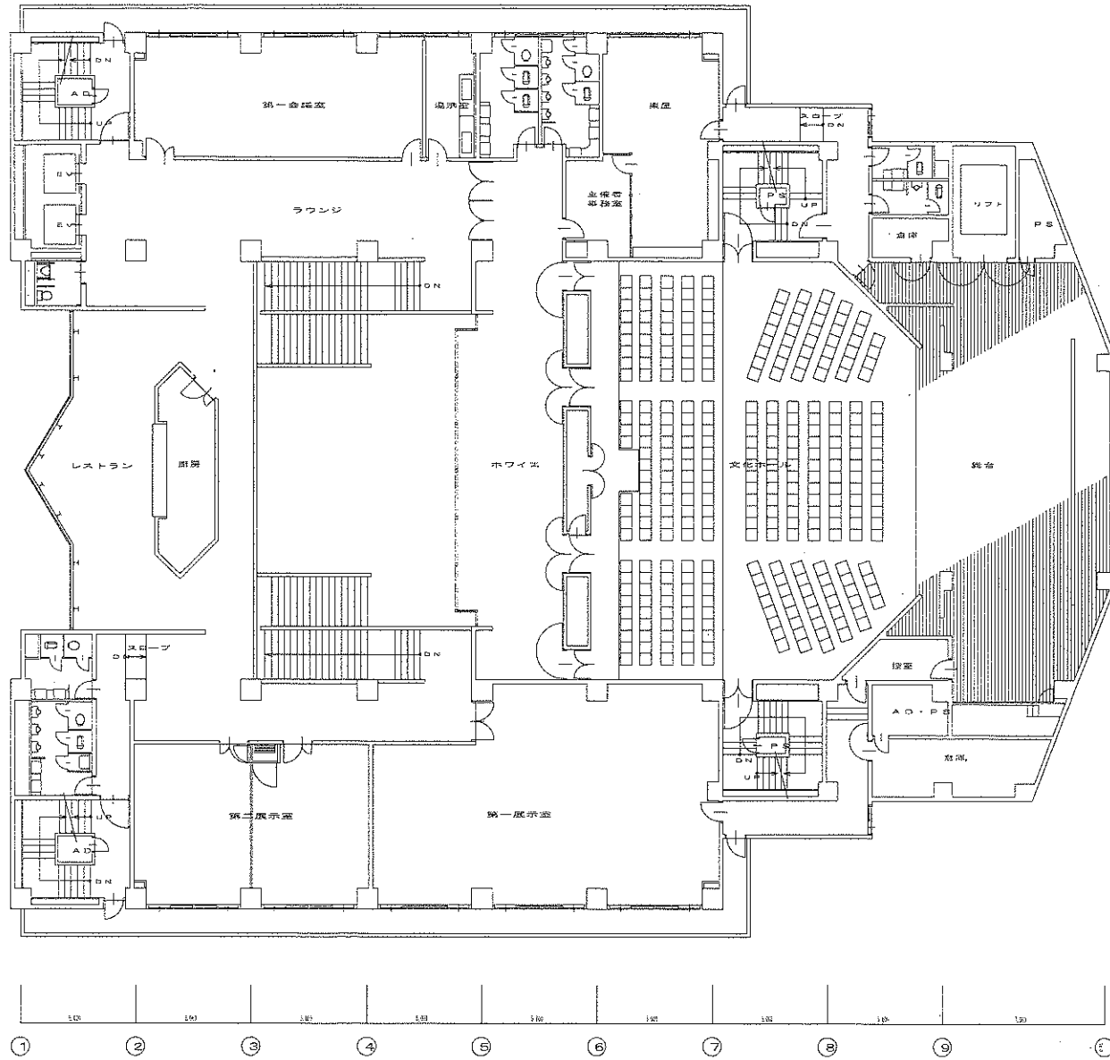
2階平面図 1:100
