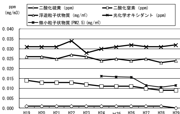
図 3-2-2 土浦保健所観測局（一般大気）における大気汚染物質（年平均値）
