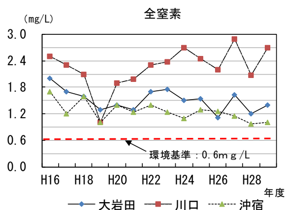
図 3-2-8 土浦沿岸の全窒素の推移
