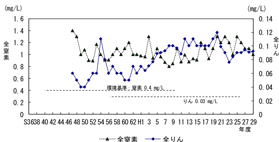
図 3-2-6 霞ヶ浦の全窒素と全リンの推移
