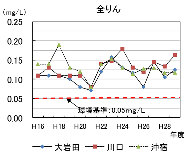
図 3-2-9 土浦沿岸の全りんの推移
