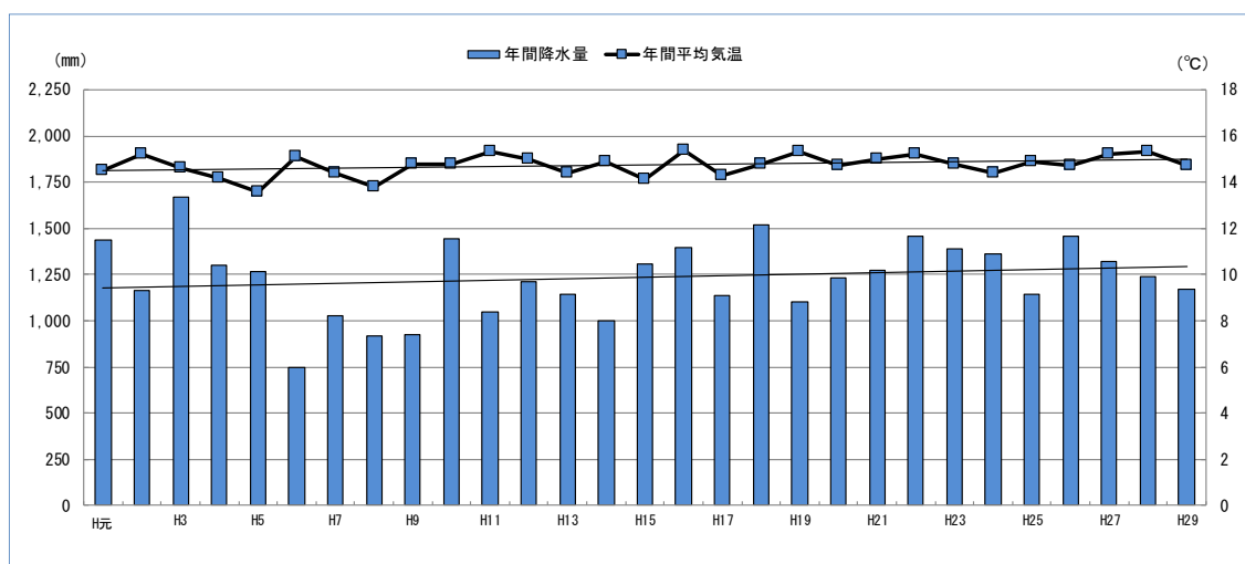
図 1-3-1 土浦観測所における年間平均気温・年間降水量の推移（気象庁）
