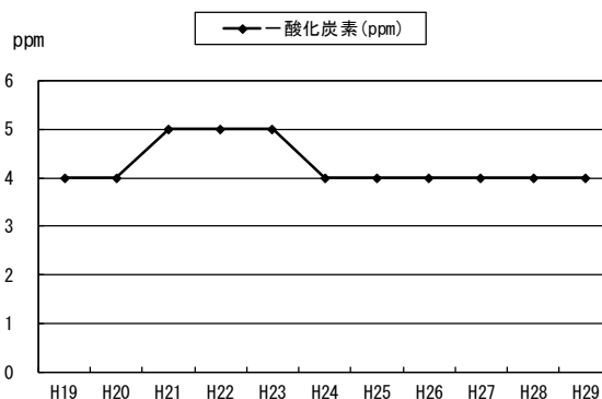
図 3-2-3 土浦中村南観測局（自動車排出ガス）における大気汚染物質
