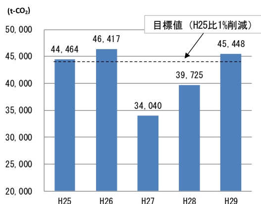
図 4-1-2 温室効果ガス総排出量実績
