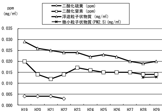
図 3-2-3 土浦中村南観測局（自動車排出ガス）における大気汚染物質
