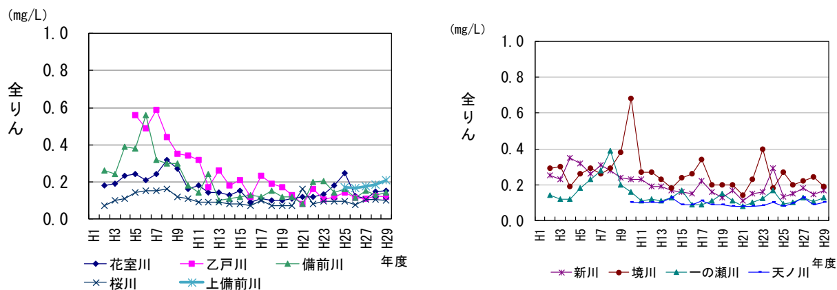
図 3-2-12 河川の全りんの推移
