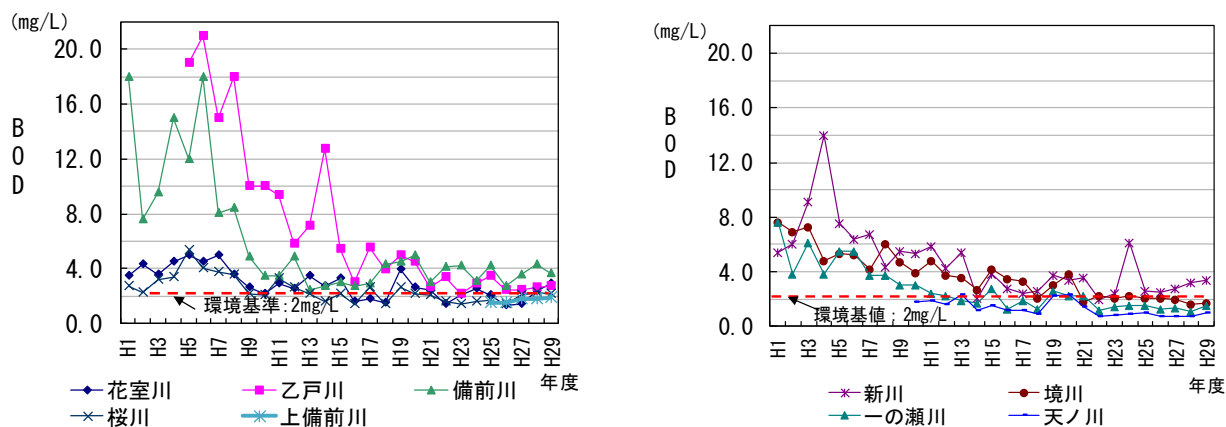
図 3-2-10 河川の BOD の推移
