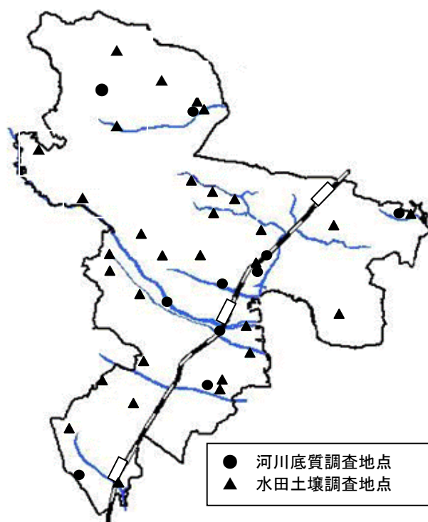
図 3-2-17 河川底質・水田土壤及び河川水質調査地点（平成 25 年度）
