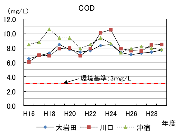
図 3-2-7 土浦沿岸の COD の推移
