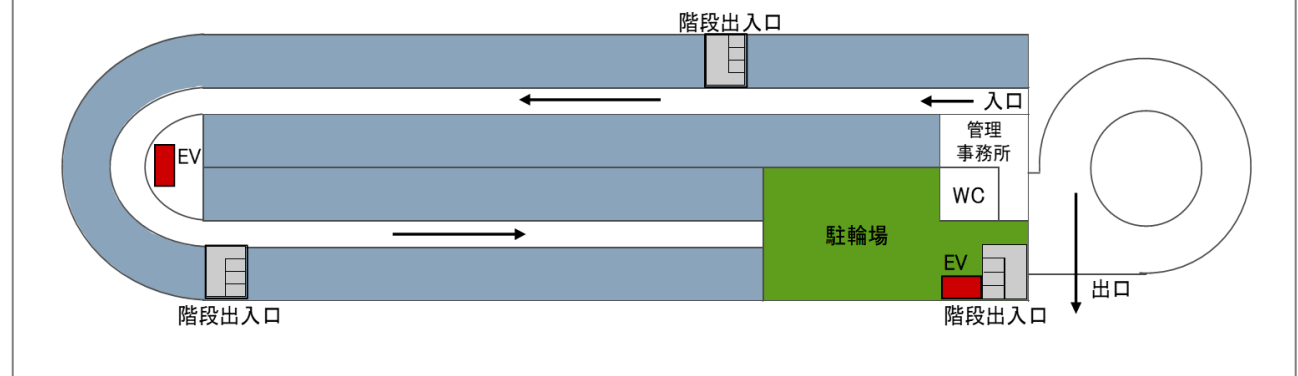
【1階平面図】
