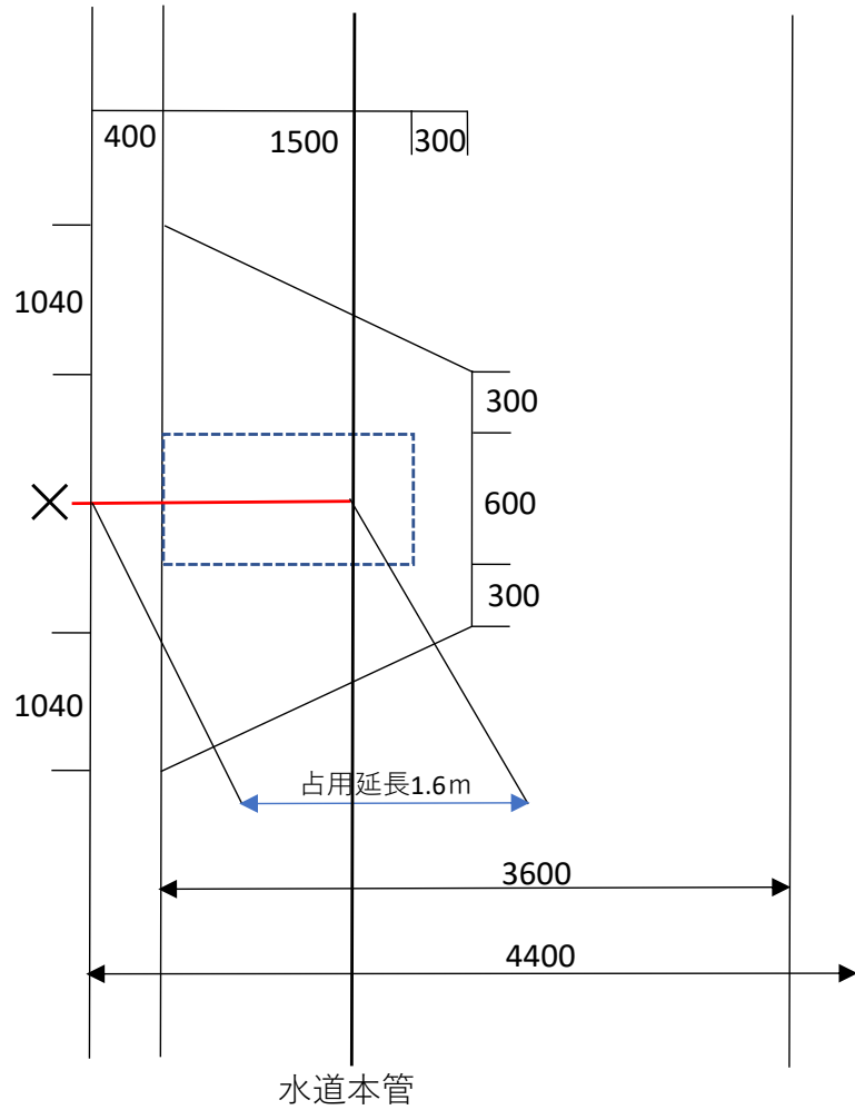
(舗装復旧平面図)
