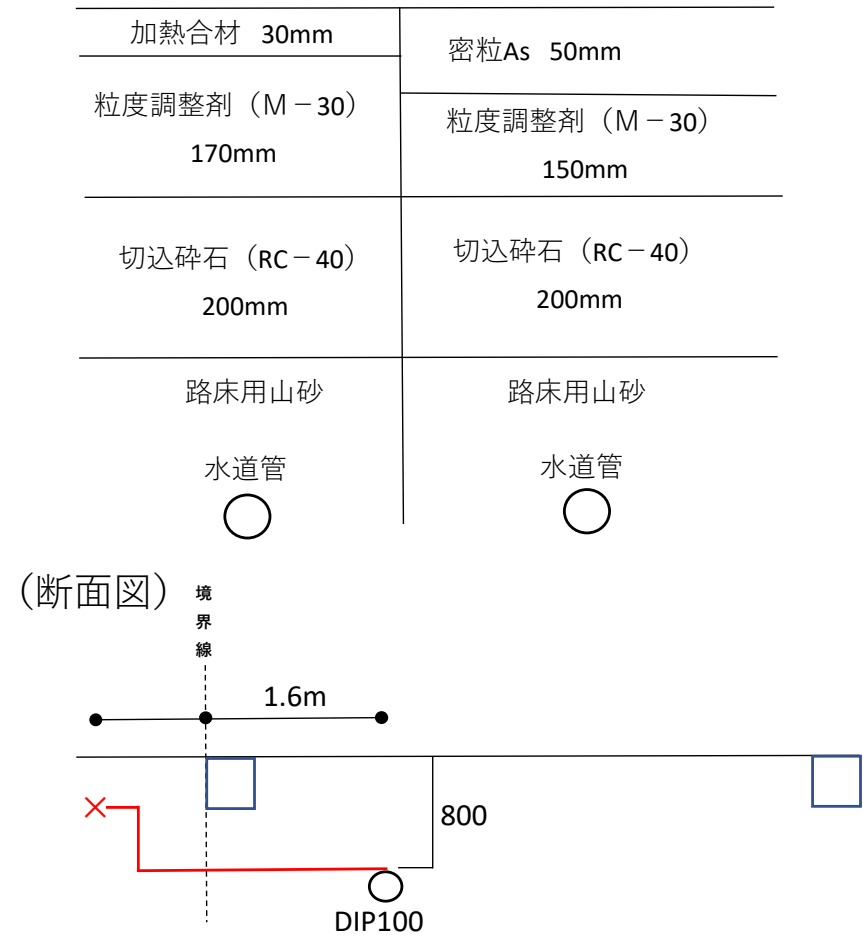
(舗装復旧断面図)
