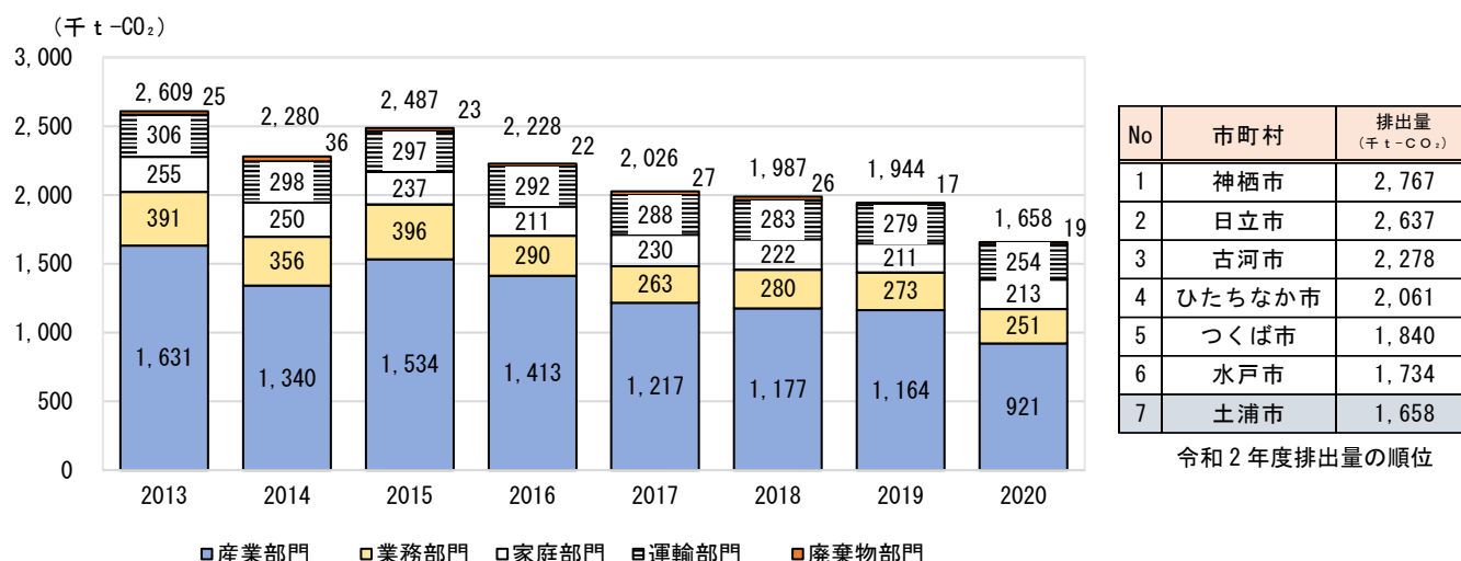
図 3-3-3 温室効果ガス排出量の推移と県内市町村比較 ※グラフ、表ともに環境省「部門別 CO 2 排出量の現況推計値」より作成
