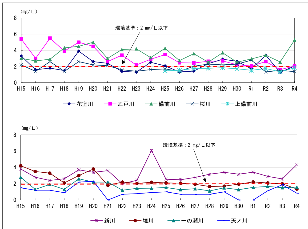
図 3-1-6 河川の BOD の推移
