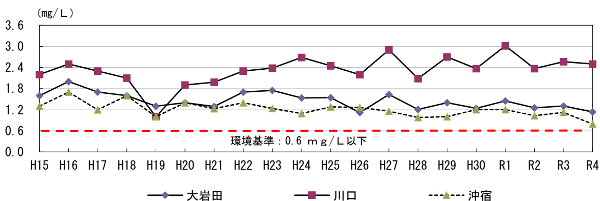
図 3-1-4 土浦沿岸の全窒素の推移
