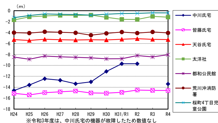
図 3-4-14 地下水位経年変化
