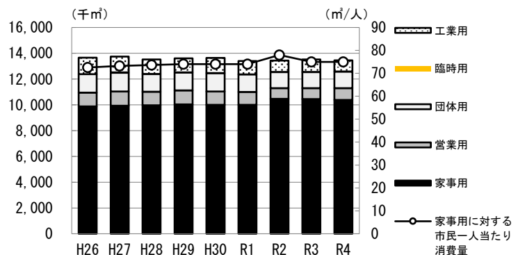
図 3-3-2 水道給水量
