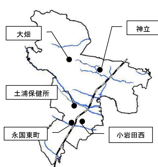
図 3-4-19 大気中ダイオキシン類測定箇所
