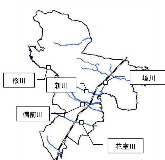
図 3-4-20 河川水及び底質ダイオキシン類測定箇所
