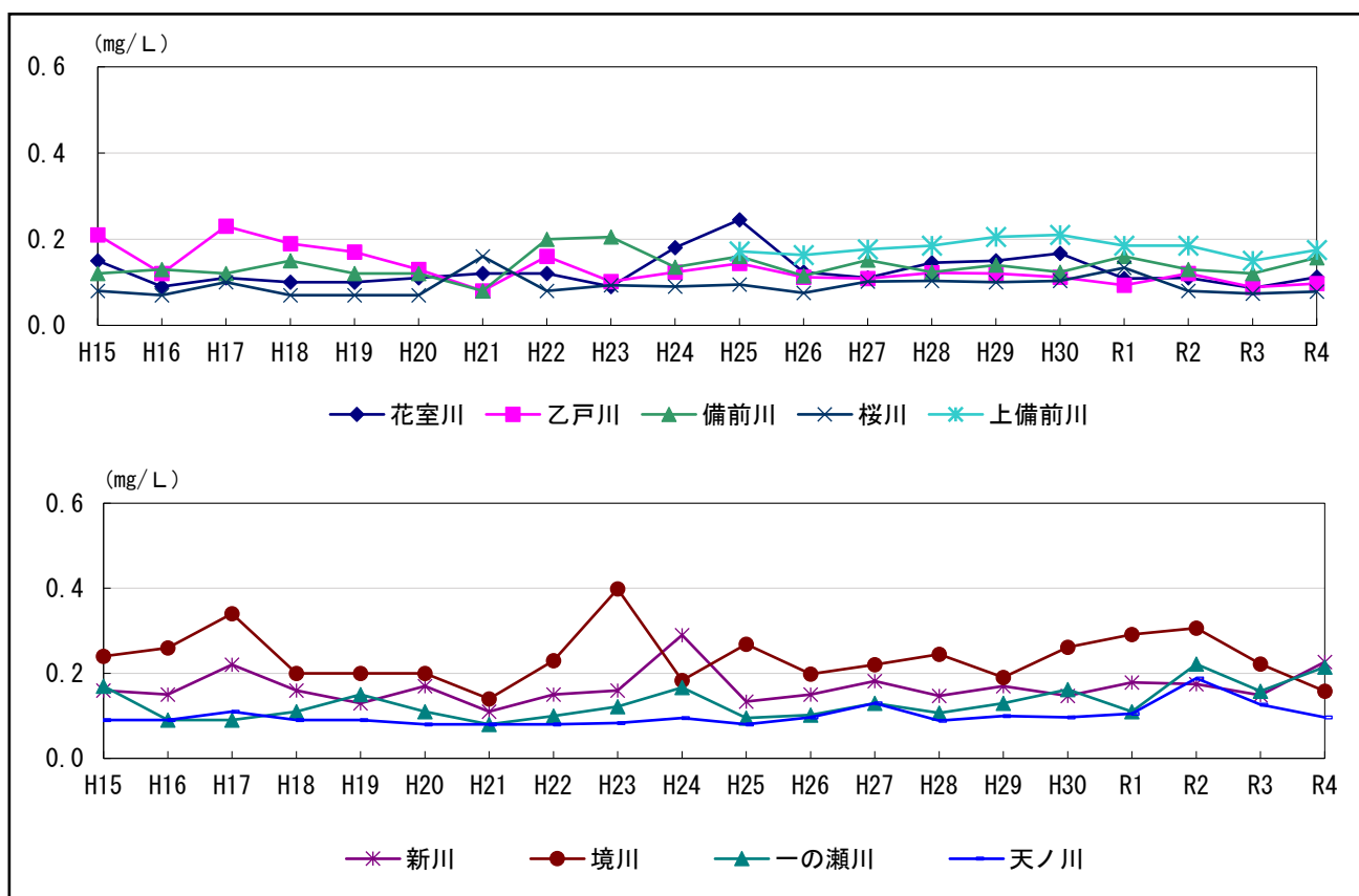
図 3-1-8 河川の全りんへの推移
