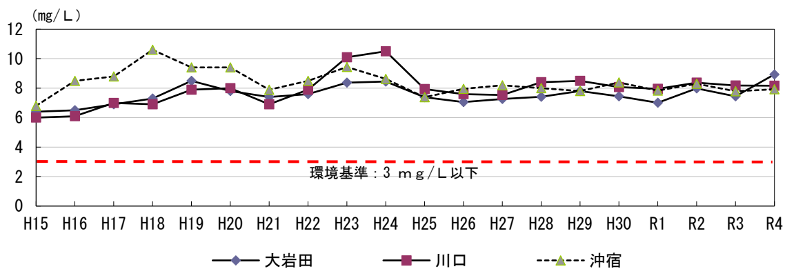
図 3-1-3 土浦沿岸の COD の推移
