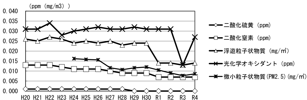
図 3-4-9 土浦保健所観測局（一般大気）における大気汚染物質（年平均値）
