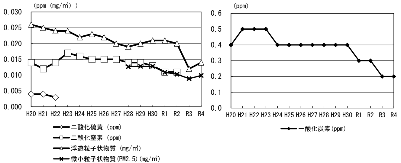
図 3-4-10 土浦中村南観測局（自動車排出ガス）における大気汚染物質
