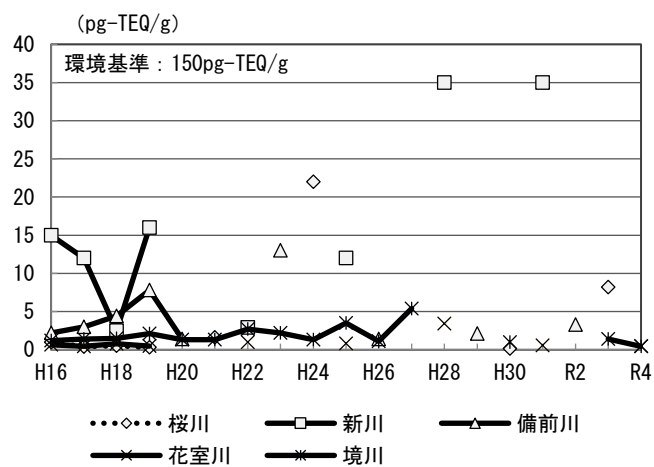
図 3-4-18 底質中のダイオキシン類測定結果（県）
