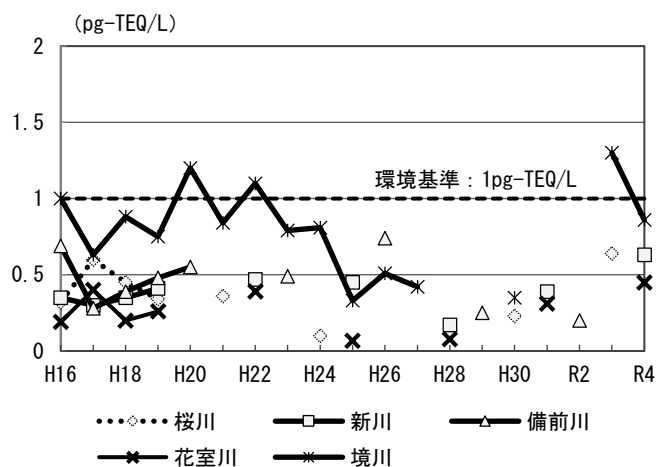
図 3-4-17 河川水中のダイオキシン類測定結果（県）
