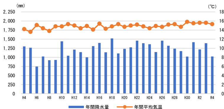
図 1-3-1 土浦観測所における年間平均気温・年間降水量の推移（気象庁）
