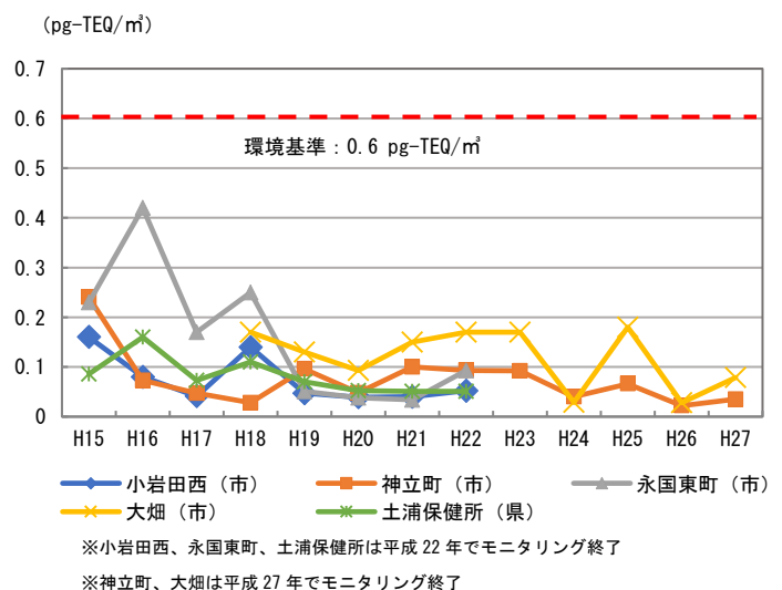
図3-4-16 大気中のダイオキシン類測定結果
