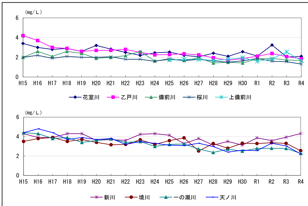
図 3-1-7 河川の全窒素の推移
