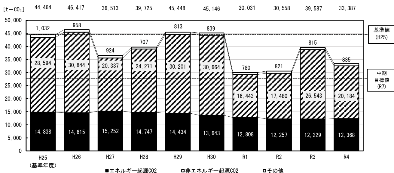
図 4-1-1 温室効果ガス総排出量実績
