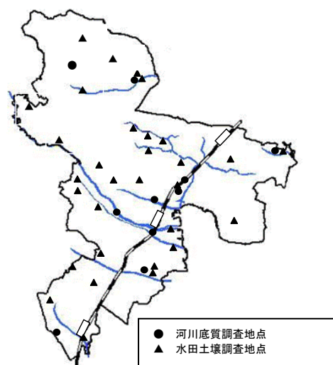
図 3-4-13 河川底質・水田土壌及び河川水質調査地点（平成 25 年度）
