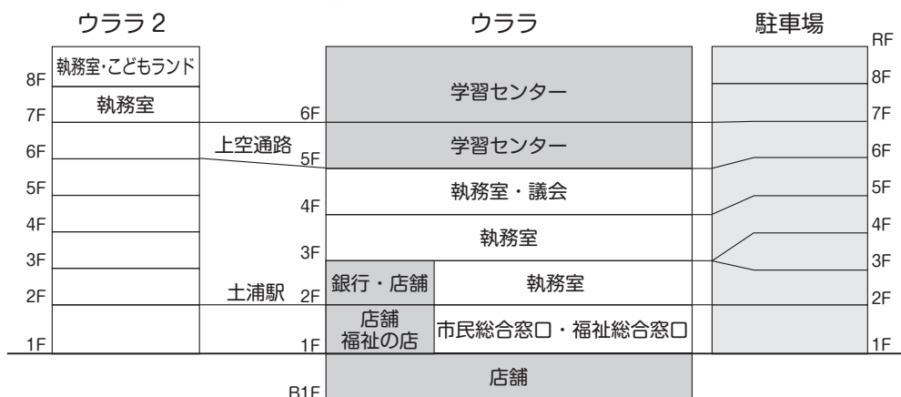
断面構成図
