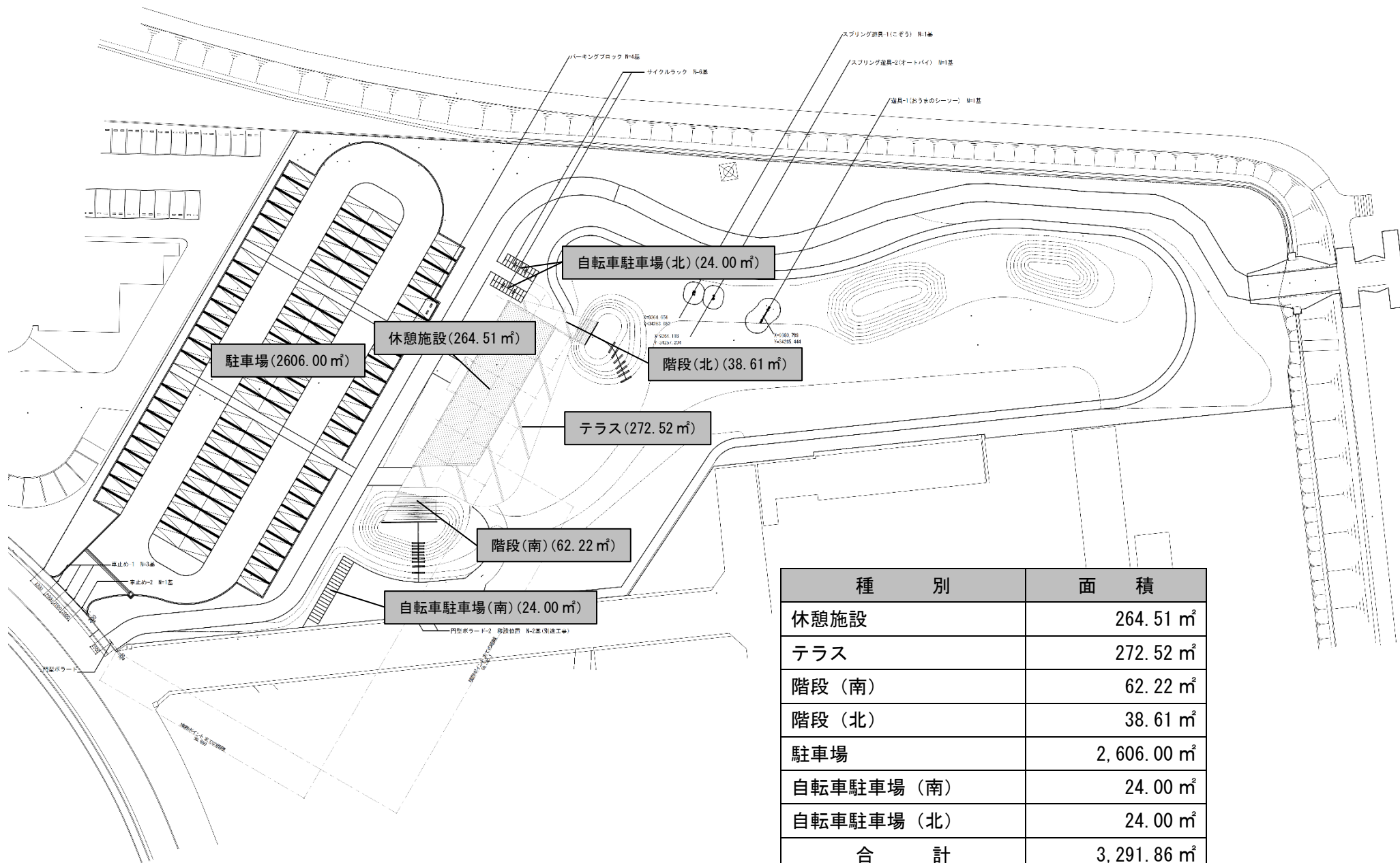
【りんりんポート土浦平面図】
