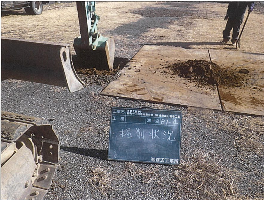
写真区分: 施工状況写真 写真タイトル: 掘削状況 撮影箇所: B1-4
