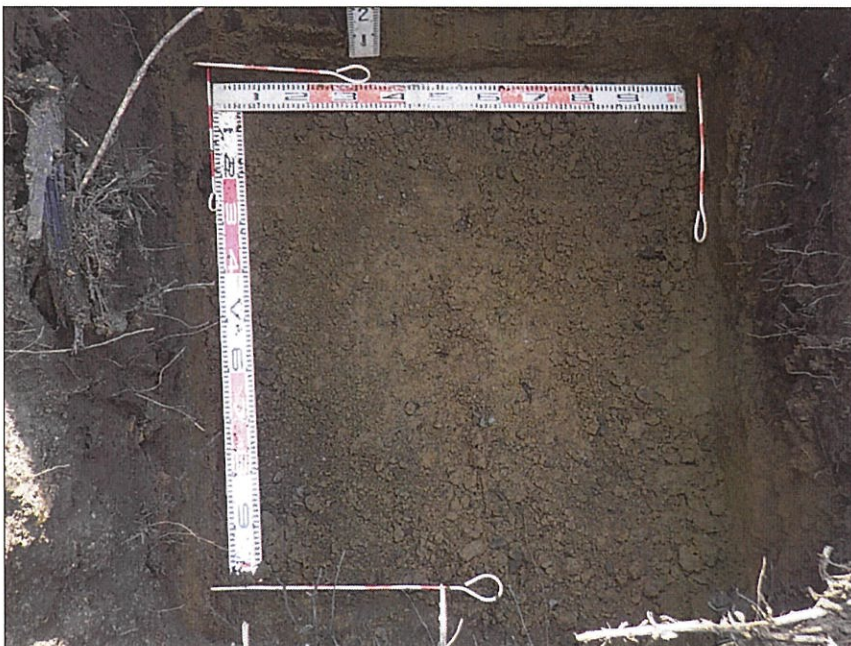
写真区分:出来形管理写真 写真タイトル:掘削出来形 撮影箇所:B1-6 施工管理値:設計H=1500 W1 =1000 W2=1000 実測H=1500 W1=1000 W2=1000
