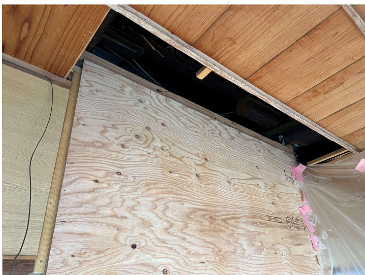
⑤ 構造補強工事(A工法)
